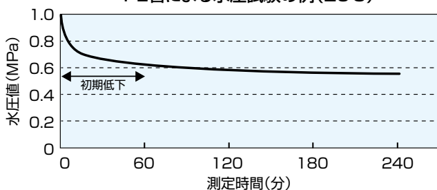
PE管による水圧試験の例(20℃)
