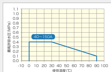
HTエスロクリーンヘッダー プラントHT(T-17)ヘッダー
