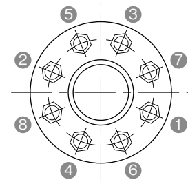
ボルト締付け順序
