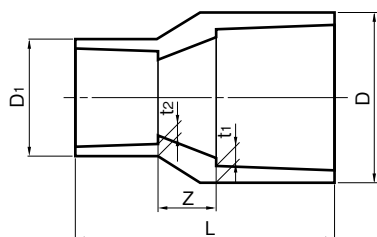
組合せ径違いソケット
