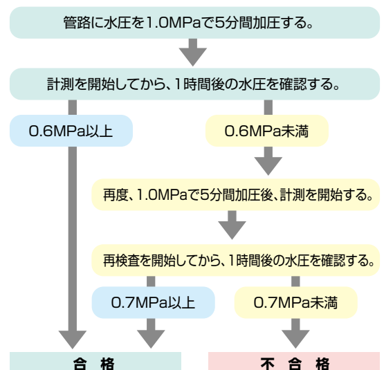
【参考：水圧漏れ試験例(20℃)】
