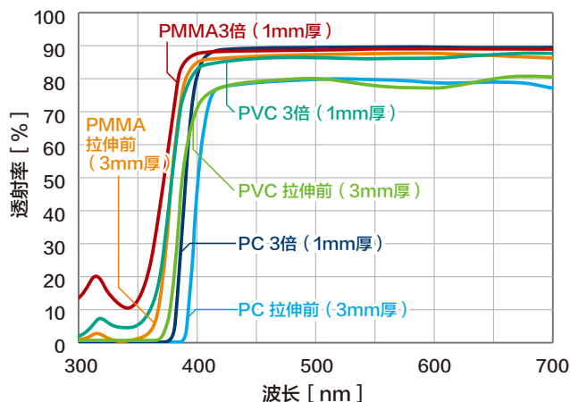
分光透射
