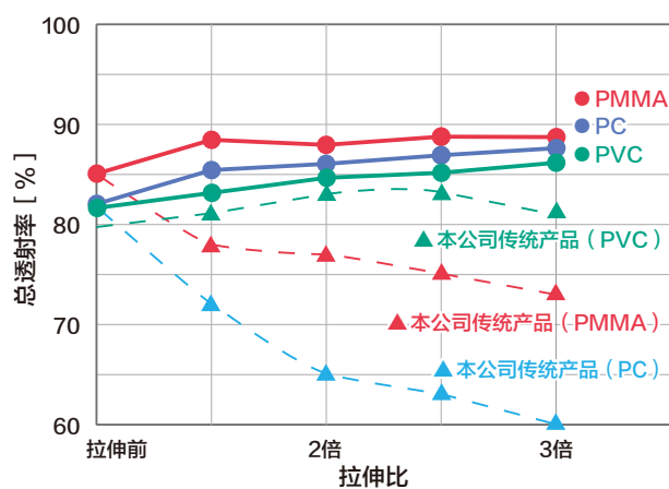
总透射率
