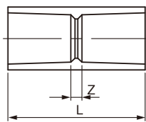
呼び径 size 20~50
