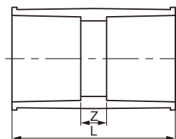
呼び径 size 65~200
