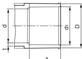
呼び径 size 65~200
