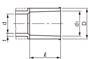
呼び径 size 20~50
