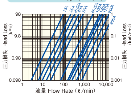
ダイヤフラムバルブ Diaphragm Valve
