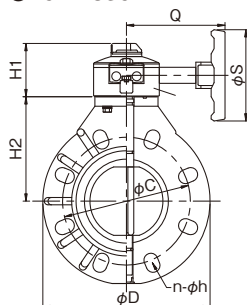
■寸法表 40A~350A Dimension Table 40A~350A
