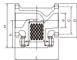
●フランジ式 Flange Type (65~100A)
