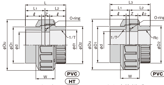
TSソケット TS Socket
