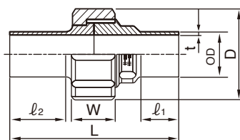
PN16 単位Unit: mm
