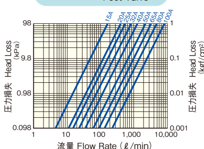
ボールチャッキバルブ Ball Check Valve フットバルブ Foot Valve
