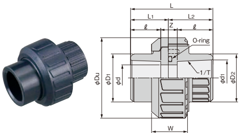
PVC(16~100), HT(C-PVC)(16~50) オリング O-ring:EPDM or FKM
