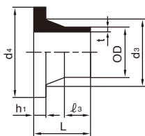
PN16 単位Unit: mm
