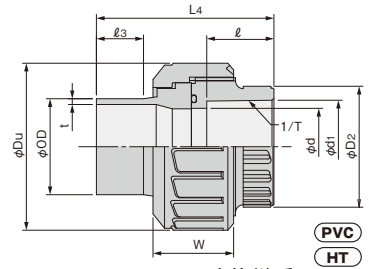
PVDF変換継手 PVDF Transtion (TS Socket-Butt)
