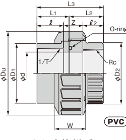
ねじ変換継手 Thread Transtion (TS Socket-Thread)
