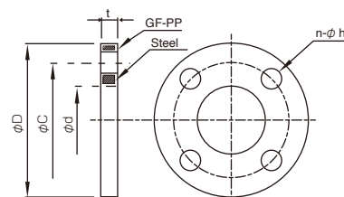
単位Unit: mm
