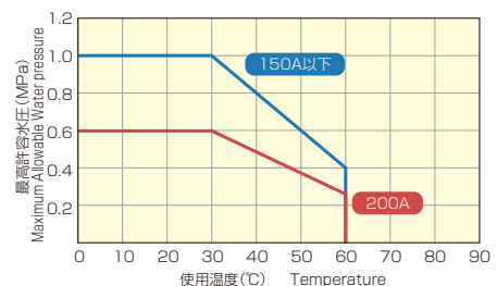
■ユニフィットの使用温度と最高許容水圧 Maximum Allowable Water Pressure-Temperature Rating
